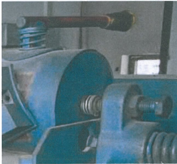
松闸顶杆（带扭簧可防止随铁芯转动）
